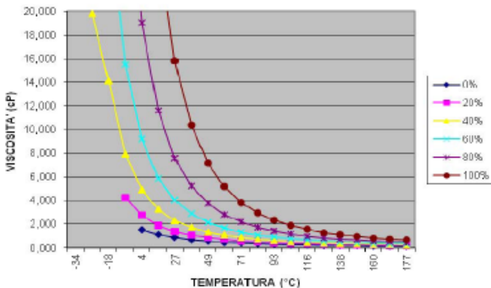
VISCOSITA' ASSOLUTA DI SOLUZIONI ACQUOSE DI ANTIFREEZE LONGLIFE BLU CONCENTRATO
