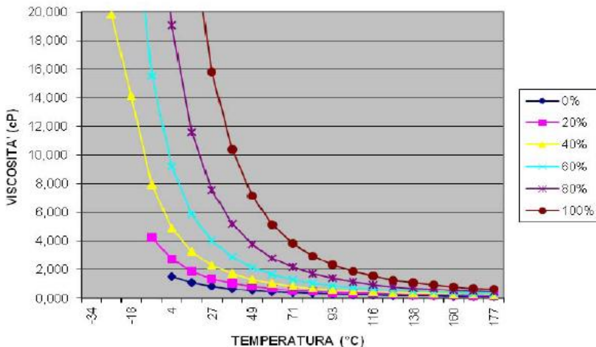
VISCOSITA' ASSOLUTA DI SOLUZIONI ACQUOSE DI LIQUIDO RAFFREDDAMENTO HOAT GIALLO
